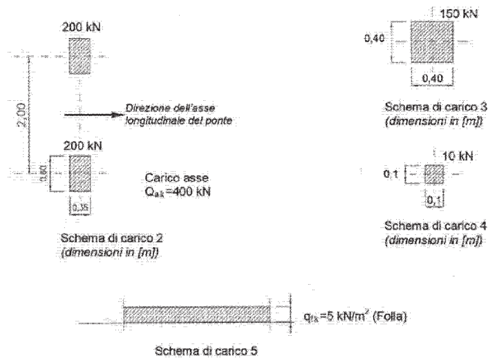
Figura 5.1.2 - Schemi di Carico 1-5 Dimensioni in [m]
