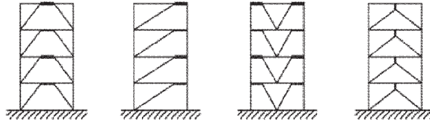
c) Strutture con controventi eccentrici
