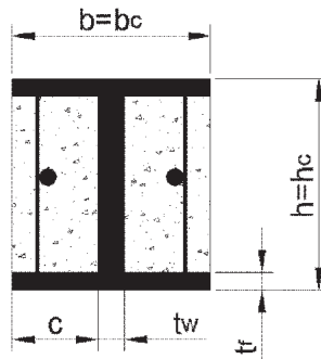
Figura 7.6.1 - Rapporti dimensionali
